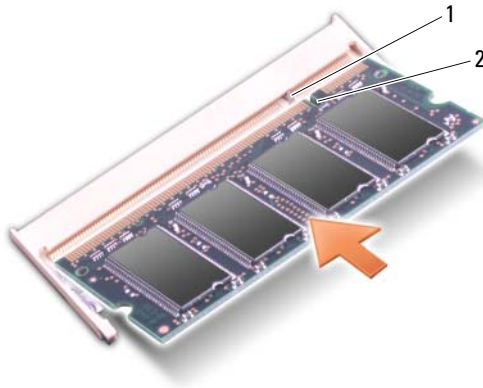
1 linguetta 2 tacca
